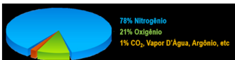
Figura 1: Composição do Ar Atmosférico
